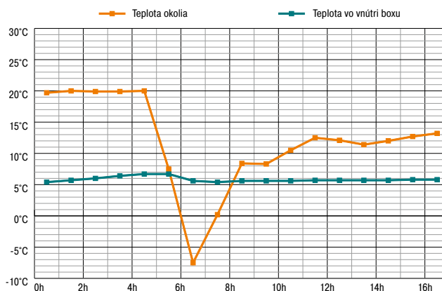
Curva di temperatura "profilo inverno" nel kit di isolamento
